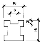
Mittel-/Eckpfosten
