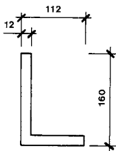
Winkelement
