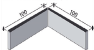
Ecke 90° 2-teilig
