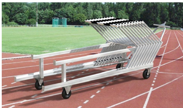
Chiot de transport de haies pour 30 haies
