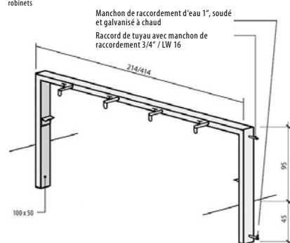
Arceau avec robinets
