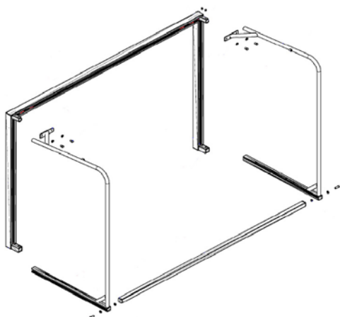
But de handball „démontable“
