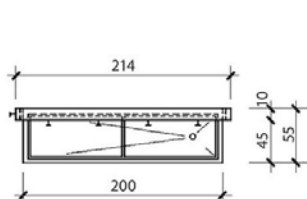
Lavoir pour chaussures type A1
