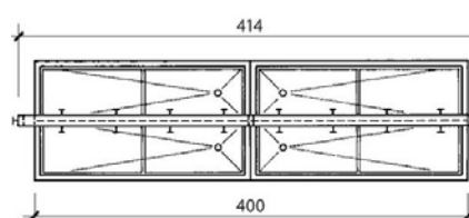
Lavoir pour chaussures type A4
