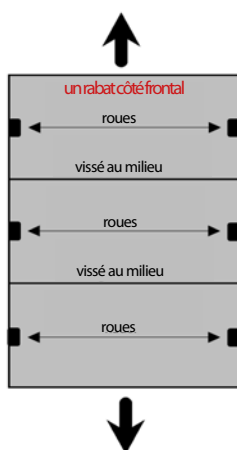
Couverture de saut à la perche „Strong” en 1 partie, abaissable, mobile vers l'arrière et l'avant
