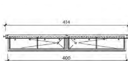
Lavoir pour chaussures type A2
