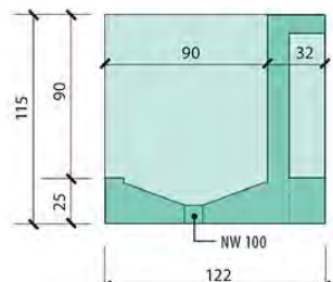
Coupe transversale exécution antigel
