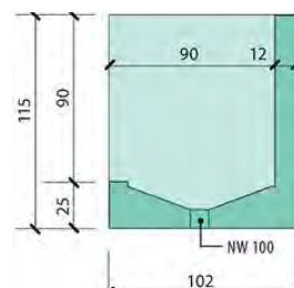
Coupe transversale exécution normale
