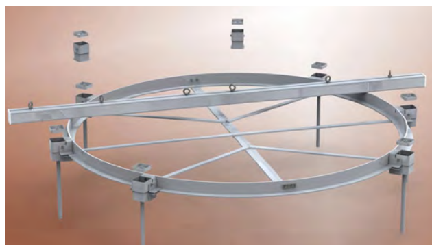
Cercle de lancer du poids adapté aux personnes handicapées, y compris deux douilles supplémentaires et une barre d'ancrage
