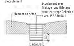
Bac de lavage : détail d'écoulement
