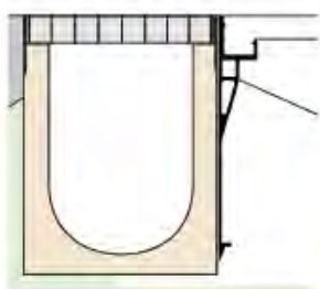
Finition sur caniveau
