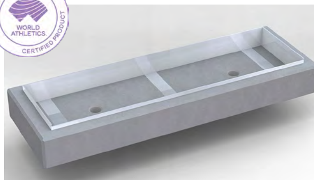
Cadre pour planche d'appel „élément en béton”
