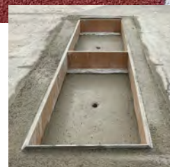
Cadre pour planche d'appel „hauteur réglable”
