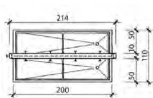
Lavoir pour chaussures type A3
