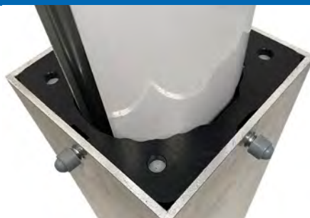
Avantage 2: Profilé de poteau en plastique guidé. Seulement 3,00cm de surface d'appui
