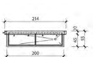
Lavoir pour chaussures type A1
