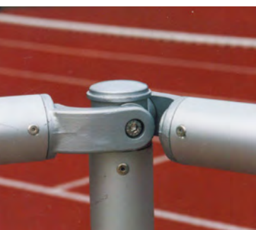
Charnière double
