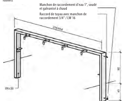
Arceau avec robinets
