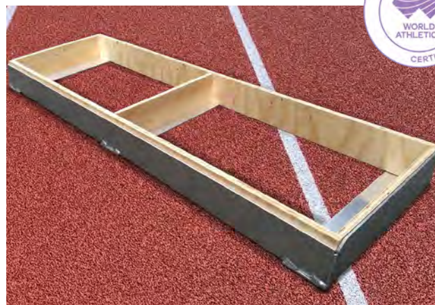
Einbauwanne „Standard“ 122/34/10 cm
