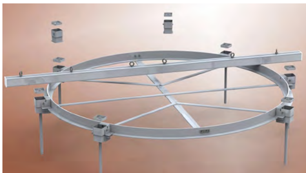
Kugelstossring behindertengerecht inkl. zwei Zusatzhülsen und Ankerbalken
