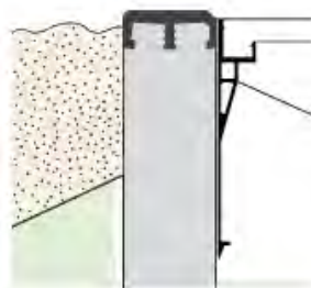
Abschluss mit Einfassung
