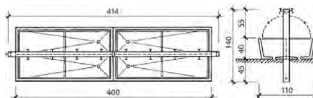
Schuhwaschanlage Typ A4
