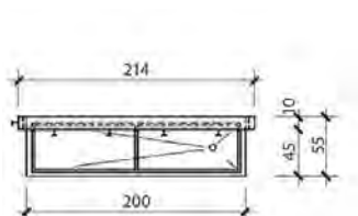
Schuhwaschanlage Typ A1
