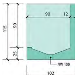
Querschnitt (Normalausführung)
