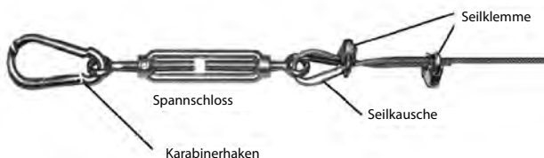
Seilklemme Art. # 4050053
