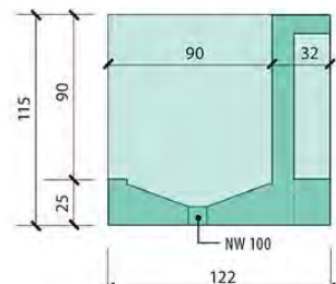
Querschnitt (Ausführung frostsicher)
