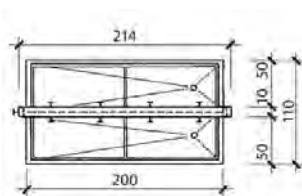
Schuhwaschanlage Typ A3
